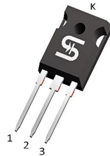
TO-247-3L
