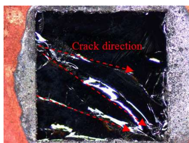
Fig 4. Die crack
